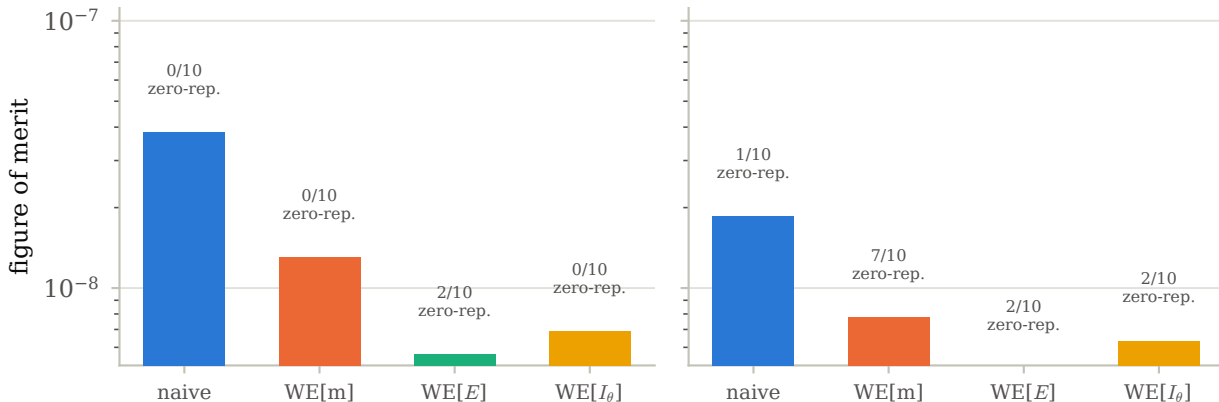
ferromagnet
